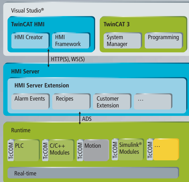
Engineering-Architektur des TwinCAT HMI
