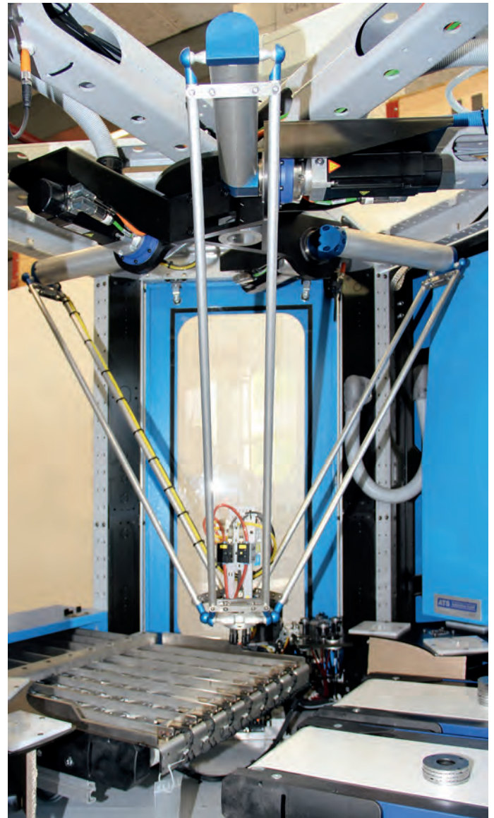
Die Steuerungs- und Antriebstechnik von Beckhoff – vom Panel-PC CP6203 bis hin zu den Servomotoren AM30xx – ermöglicht einen dynamischen Delta-Roboter und damit einen schnellen und präzisen Prüfablauf.
